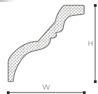
TL NOMASTYL® PLUS H 150 x W 150 mm
