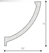
L3 ARSTYL® H 175 x W 145 mm p33
