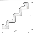
TI NOMASTYL® PLUS H 140 x W 140 mm
