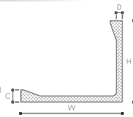
L5 ARSTYL® H 200 x W 200 mm C 27 mm - D 15 mm p33
