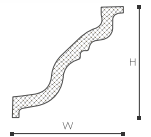
TL NOMASTYL® PLUS H 150 x W 150 mm
