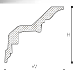
Z6 ARSTYL® H 120 x W 125 mm
